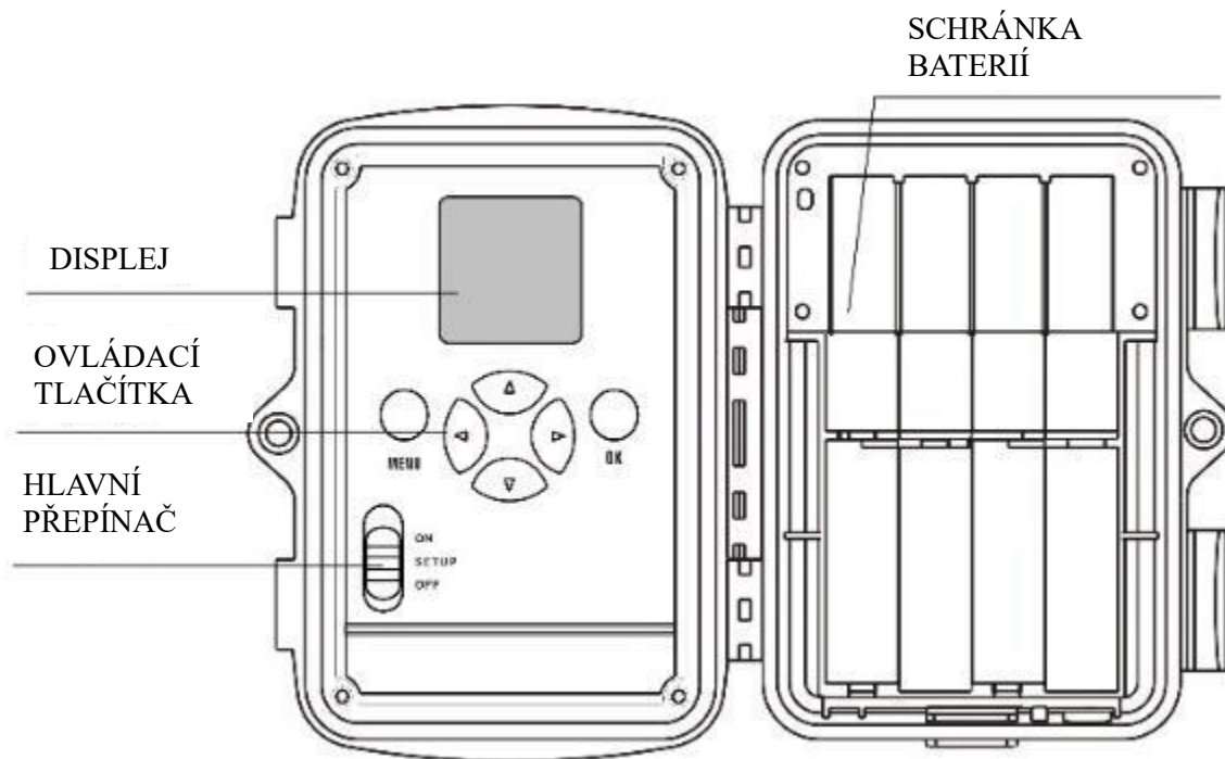
Obr. 1: Pohled zředu
