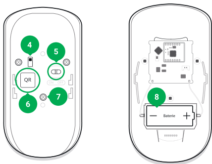
4 - Sabotážní kontakt 5 - Přepínač pro vypnutí / zapnutí 6 - QR kód 7 - Vrutky pro zajištění krytu detektoru
