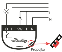
Zapojení pro napájení: 12 V a 24-60 V ss
