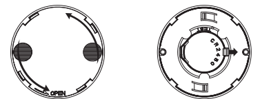
(1) Forgassa el az intelligens kulcs hátlapját és távolítsa el. (2) Vegye ki és cserélje le 1x CR2450 akkumulátorra.
