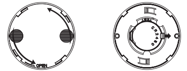
(1) Otočte zadný kryt chytrého tlačítka a odstráňte ho. (2) Vyberte a vyměňte za 1x batériu CR2450.
