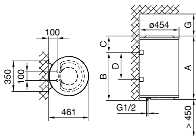
Obr. 1: Svislá instalace na stěnu
