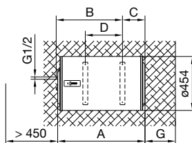
Obr. 2: Vodorovné umístění na stěnu
